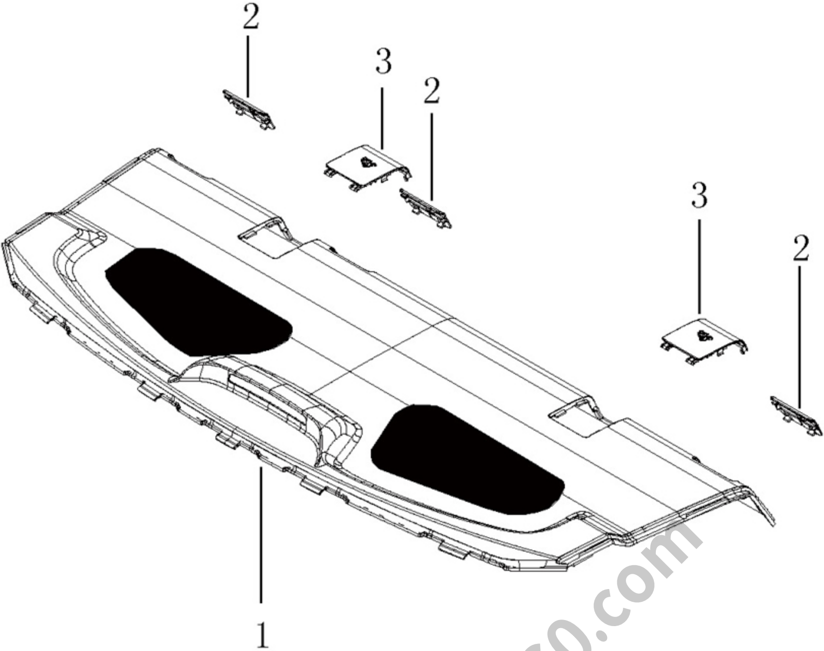
后窗台装置视图
